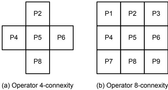
Gambar 3. 2 jenis operator lokal pixel
