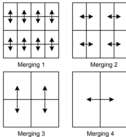
Gambar 8. Algoritma paralel O(n) pada arsitektur 2D Polymorphic-Torus
