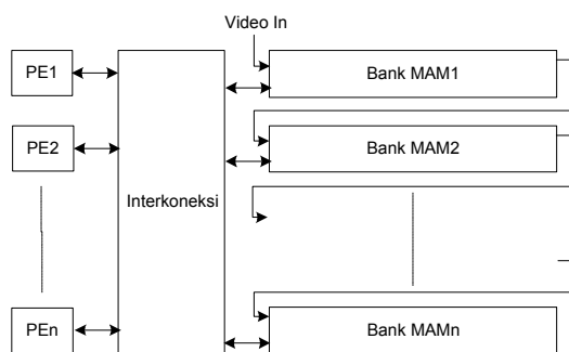
Gambar 9. Model arsitektur paralel yang digunakan
