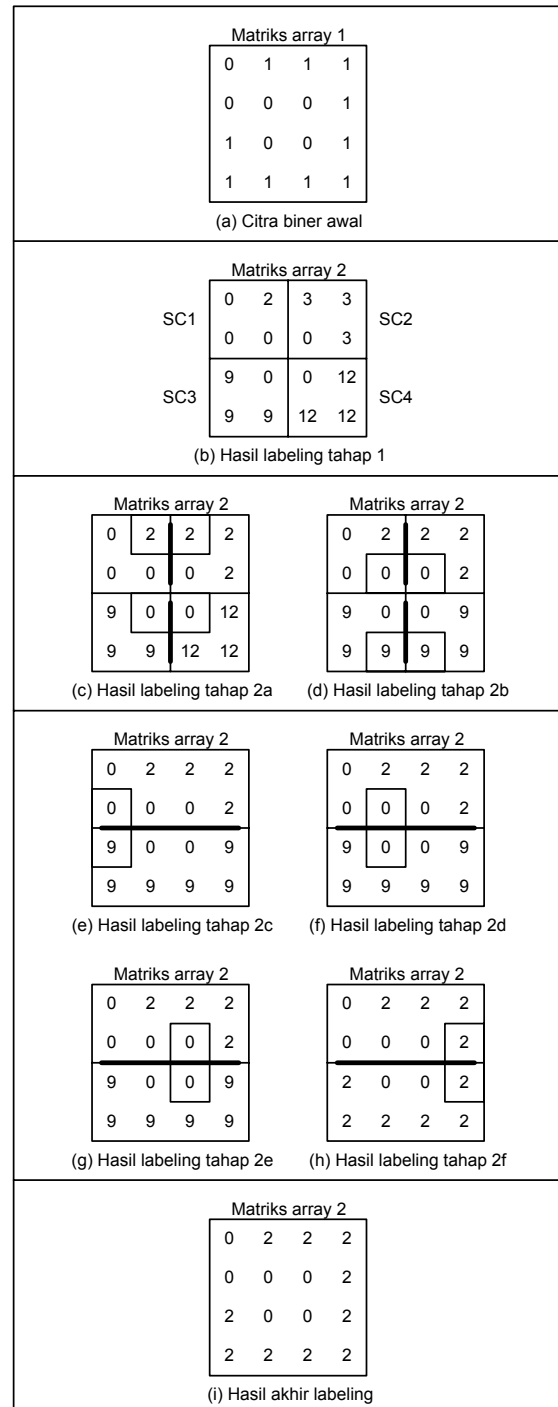
Gambar 10. Ilustrasi labeling optimal Processor-Time O(n) yang diusulkan pada struktur array berdimensi 2
