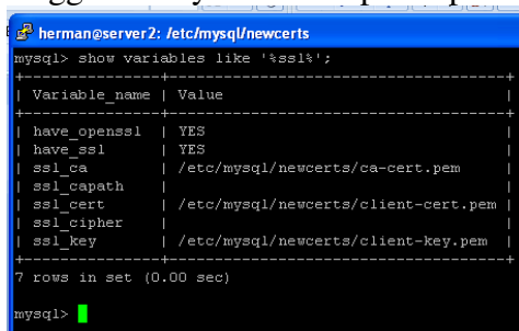
Gambar 6. Hasil Konfigurasi certificate authority SSL Untuk Server Slave
