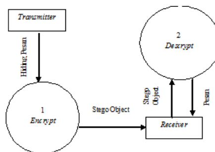
Gambar 2. DFD Level 1
