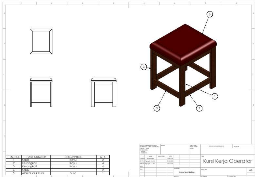
Gambar 8. Gambar Proyeksi Orthogonal Alat Pemotong Cantel Aluminium dan Kursi
