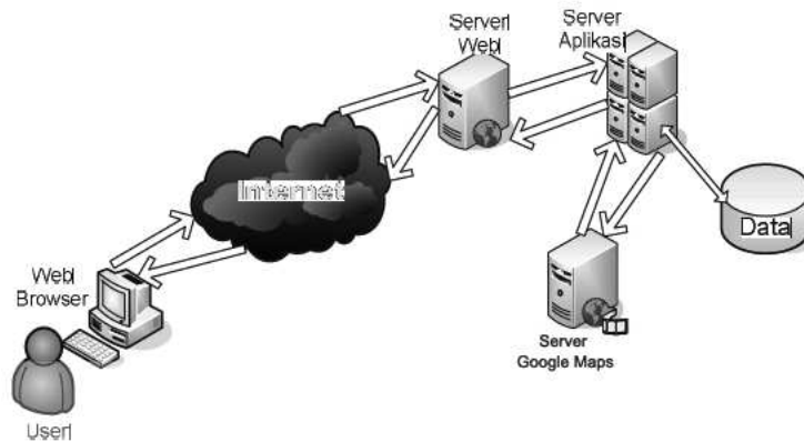
Gambar 1. Arsitektur SIG Berbasis Web.
