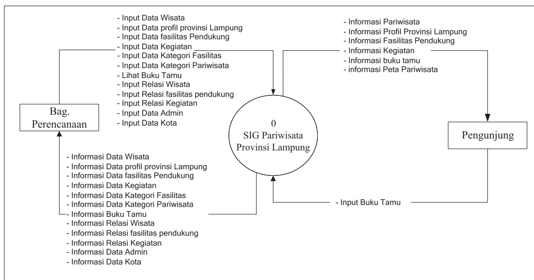
Gambar 2. DFD Level 0 Sistem Informasi Geografis Pariwisata Provinsi Lampung.
