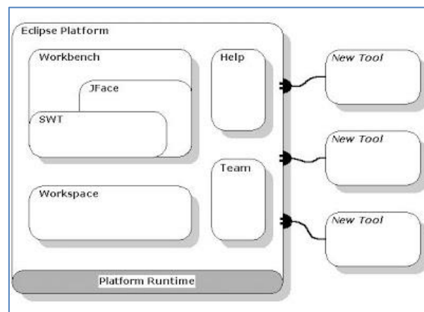
Gambar 1. Arsitektur Eclipse
