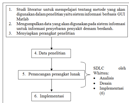
Gambar 3 Desain Penelitian
