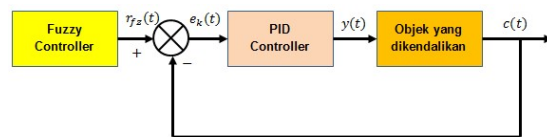
Gambar 10. Struktur Algoritma Pengendali Nitrat Berbasis Fuzzy-PID
