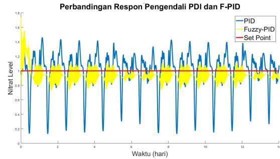
Gambar 13. Grafik Perbandingan Umpan Balik Nitrat Pada Pengendali Berbasis PID dan Fuzzy-PID
