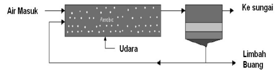
Gambar 2. Siklus Nitrifikasi di Tangki Aerasi
