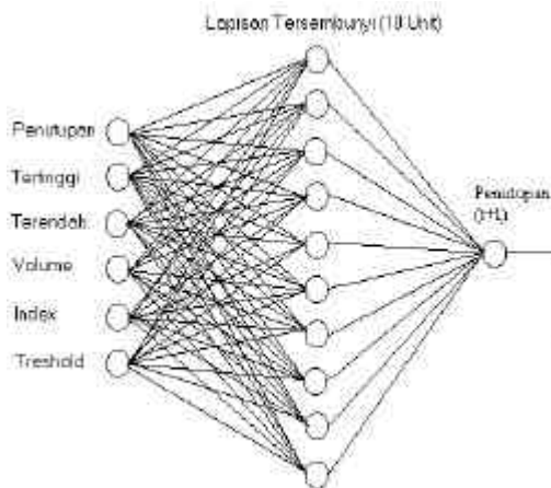
Gambar 1. Jaringan Syaraf Tiruan Feedforward Untuk Prediksi Harga saham
