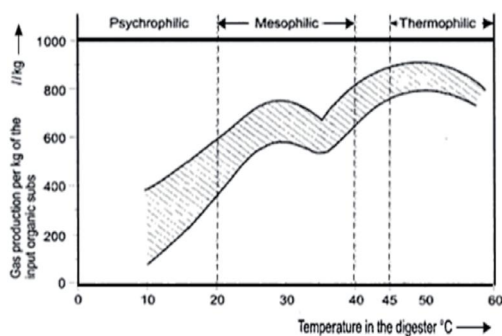
Gambar 1. Potensi Produksi Biogas Berdasar Suhu (Bouille dan Dubois, 2004)
