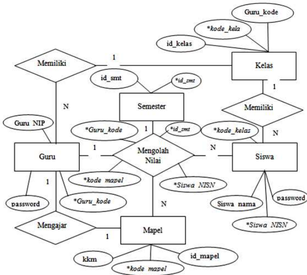
Gambar 4. ERD
