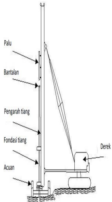
Gambar- Peralatan pemancang Pondasi tiang
